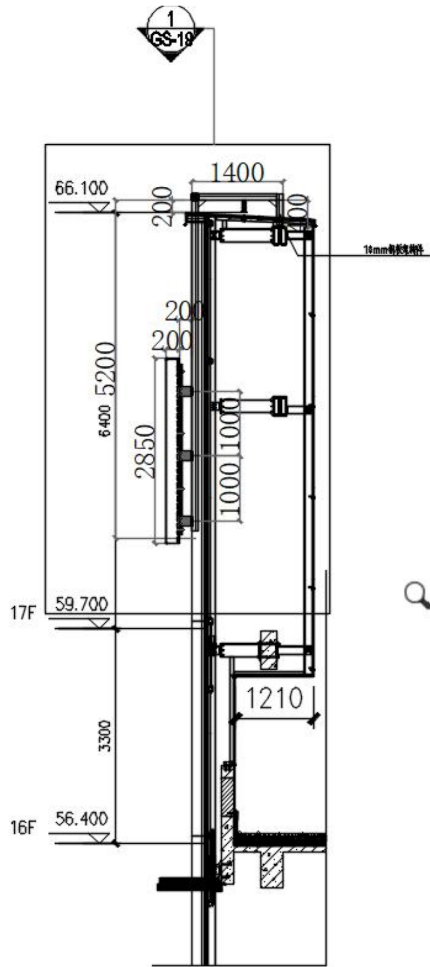
剖面图1-1
