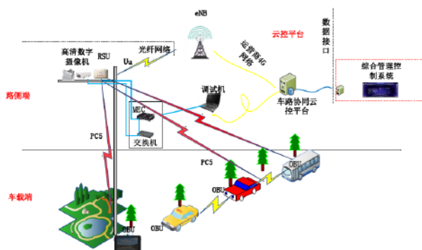
图 6.7—5 车路协同系统架构图
