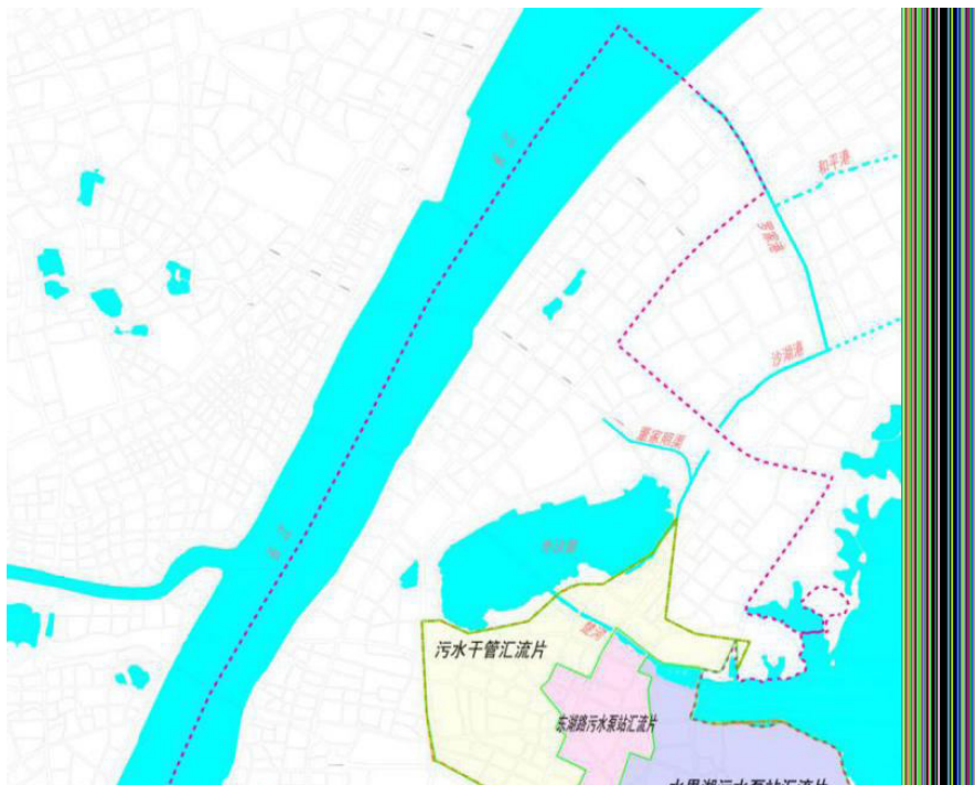
黄家湖污水收集系统现状管网布局图
