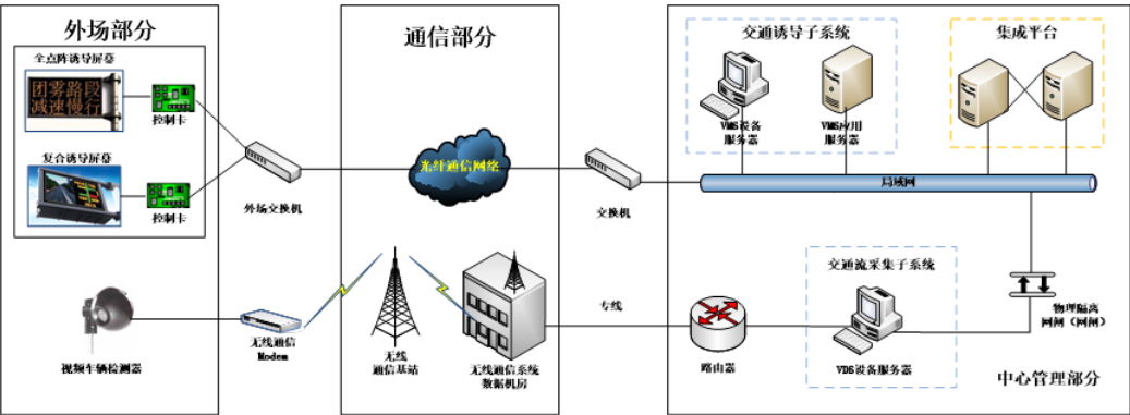
图 5-12 交通诱导数据流程
