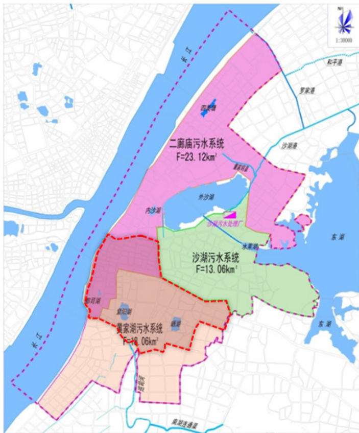
武昌区不同排水体制分区示意图
