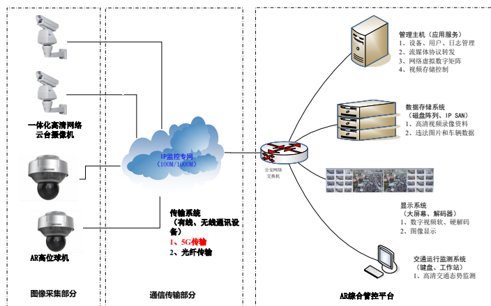
图 5-5 交通运行监测系统
