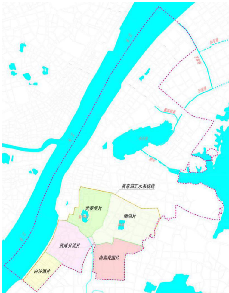
黄家湖污水系统现状分区图
