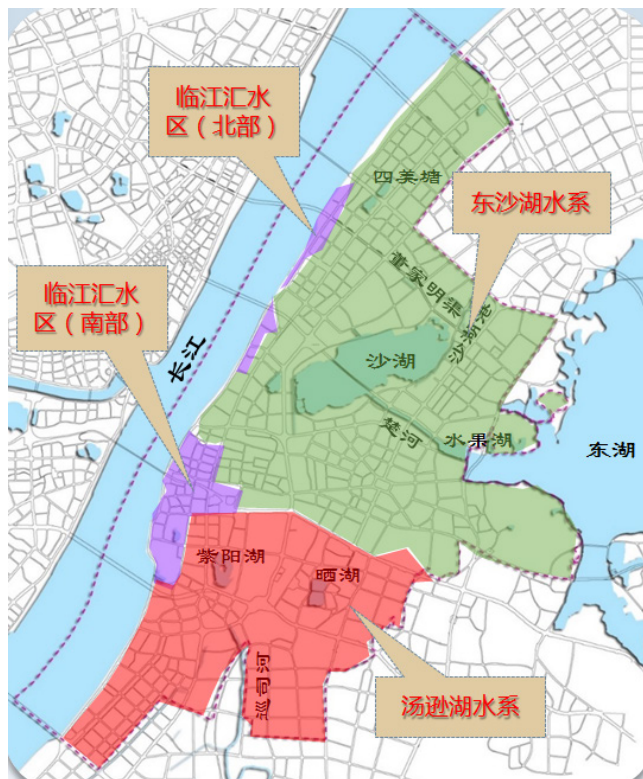
武昌区现状雨水系统分区图
