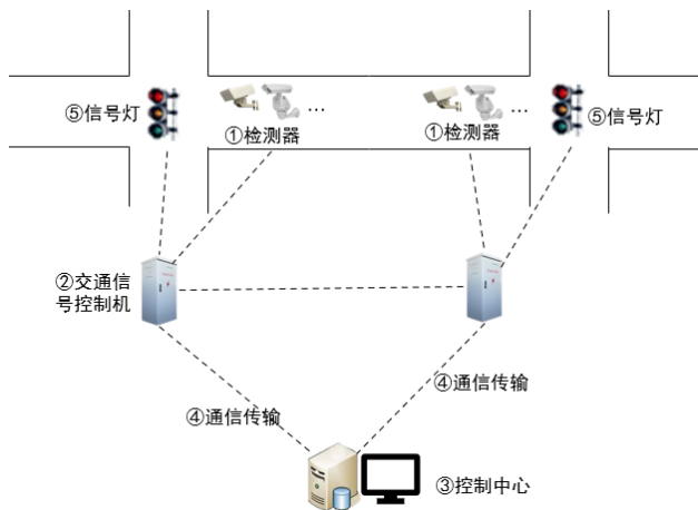
图 5-6 交通信号控制系统总体架构图
