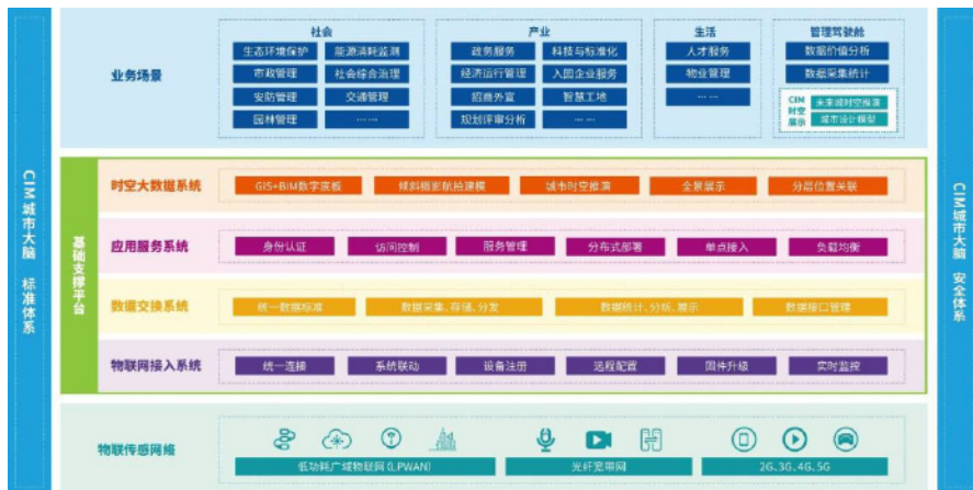
图 6.7—15 城市信息模型（CIM）平台架构图
