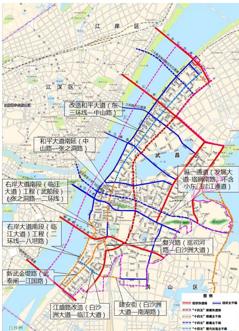
图 6.4—1 “十四五”武昌区范围内主干路建设项目分布图
